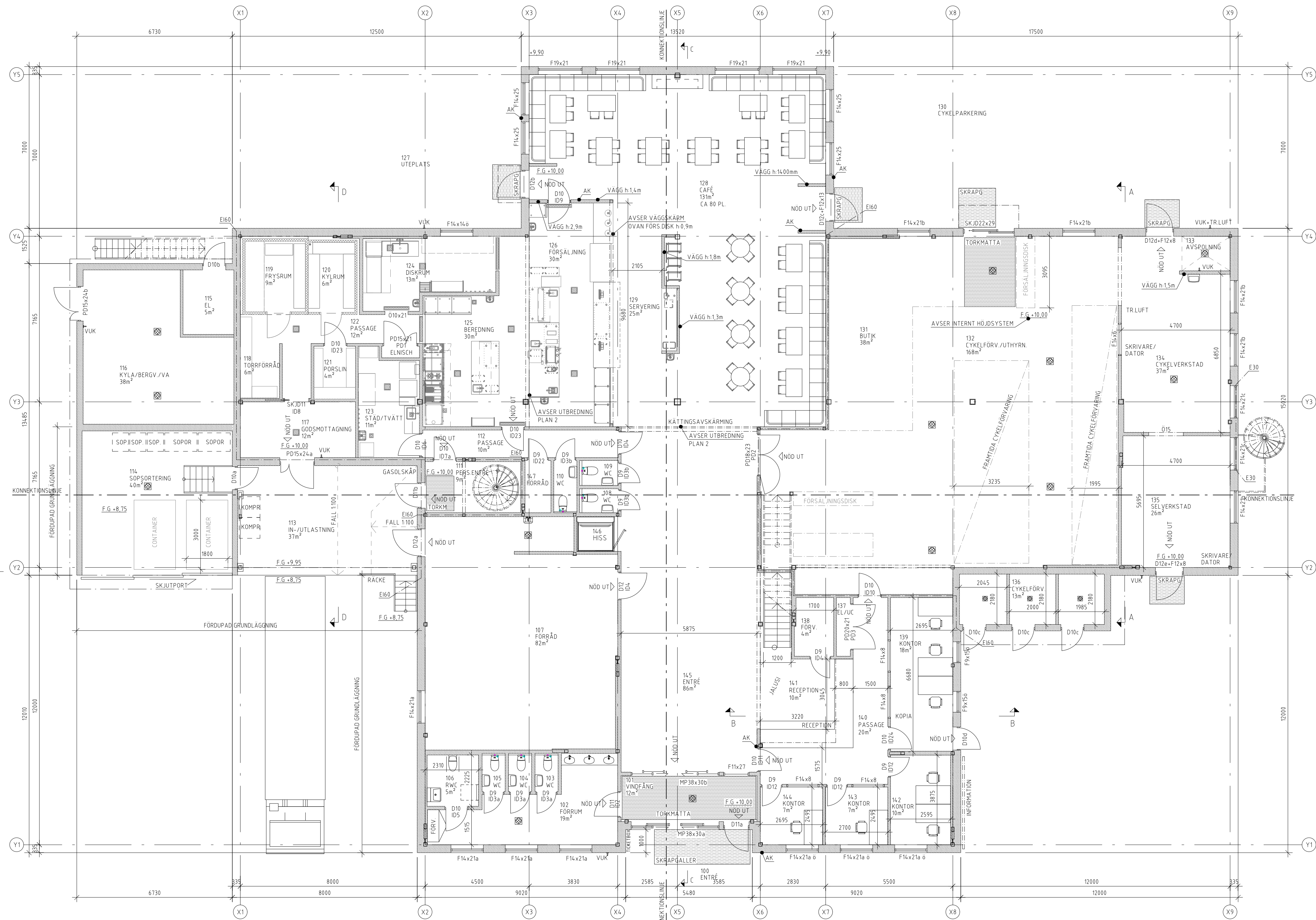
-PLAN 1, ÖVERSIKT -1:100- (A1)
